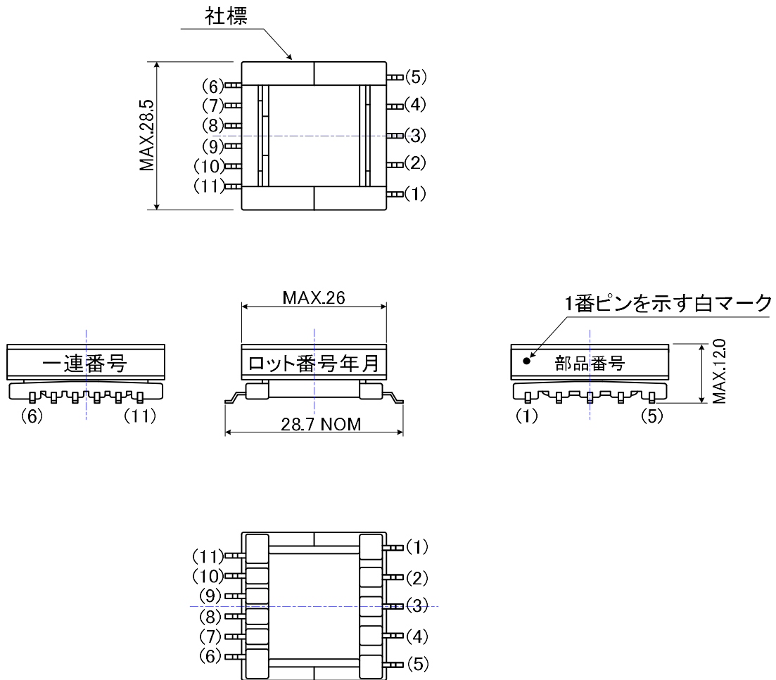
図 1 外形寸法、表示
