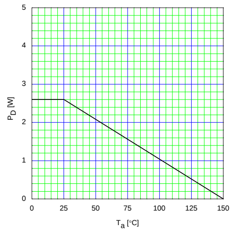
図 6 許容損失 P D – 周囲温度 T a
