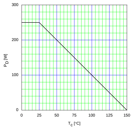
図 14 許容損失 P D – ケース表面温度 T c
