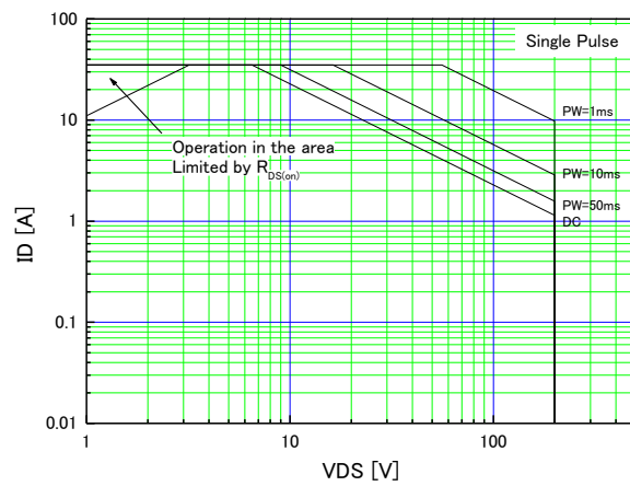
図 22 安全動作領域
