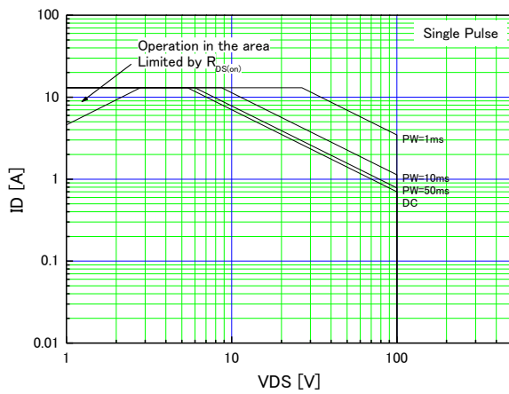
図 19 安全動作領域
