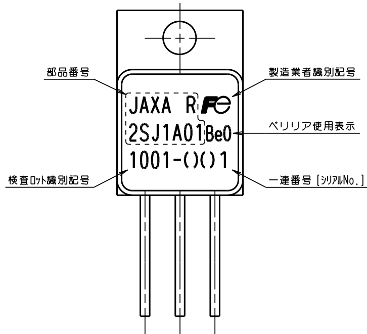
図 2a 表示内容 (TO-254) (JAXA R 2SJ1A01, 2SJ1A07)
