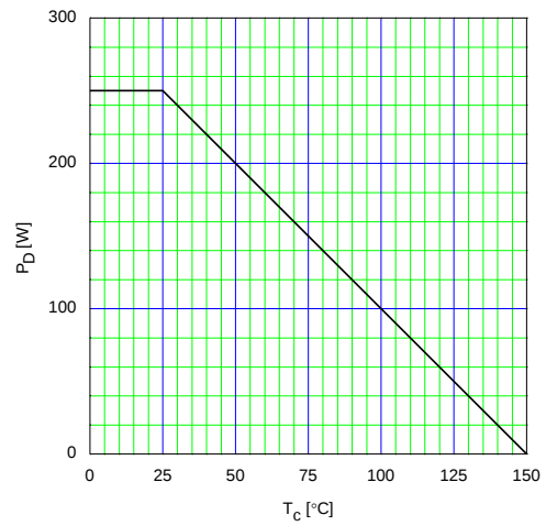
図 20 許容損失 P_D – ケース表面温度 T_c
