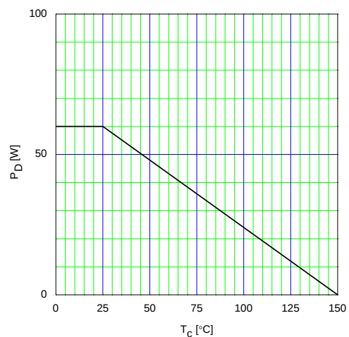
図 18 許容損失 P D – ケース表面温度 T c
