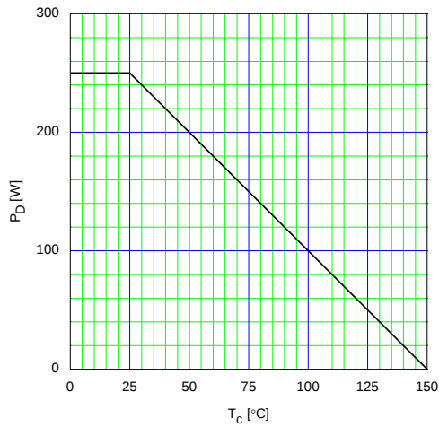
図 5 許容損失 P D – ケース表面温度 T c
