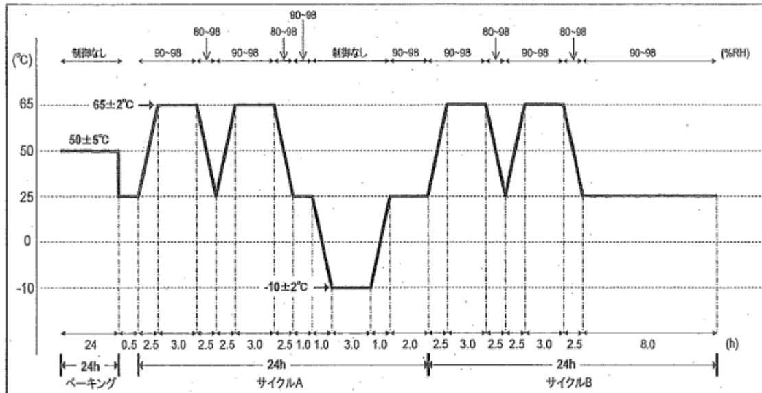
図-7 タイプⅡ湿度試験サイクル
