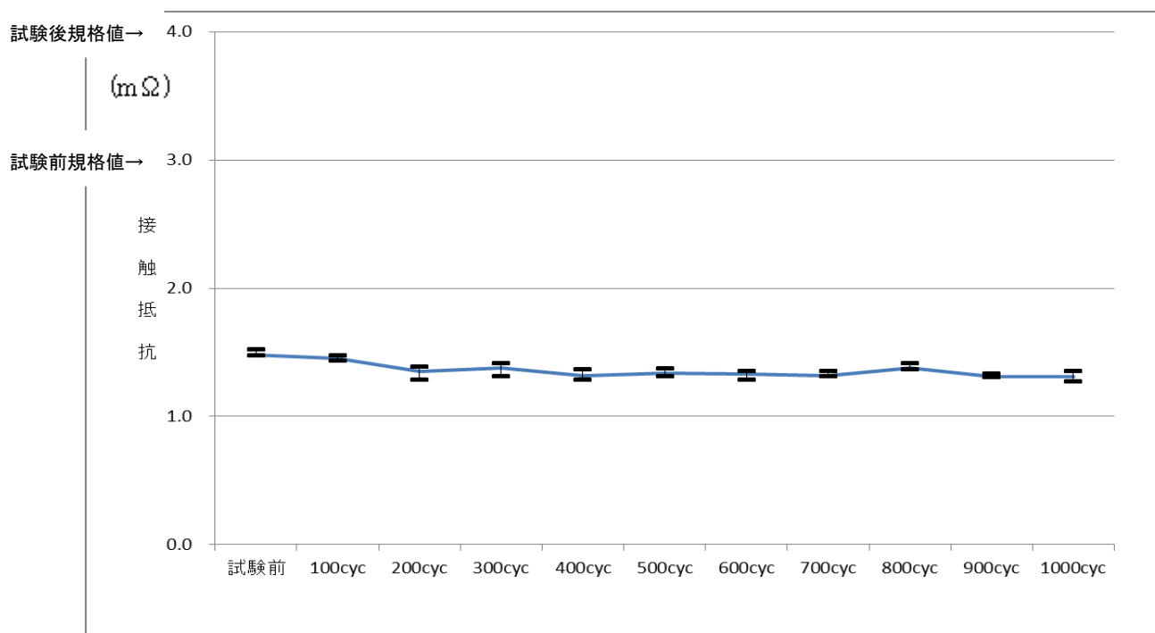
図-9 熱衝撃試験の接触抵抗
