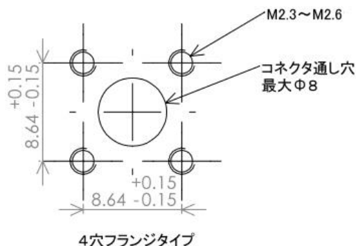
図-4 取付穴寸法
