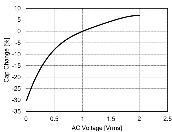
⑥2012X7SB106KS
