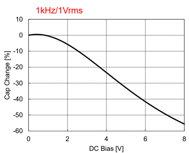
⑥2012X7SB106KS
