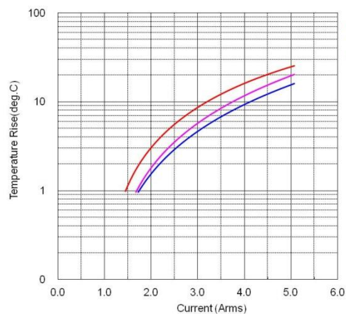
⑥2012X7SB106KS
