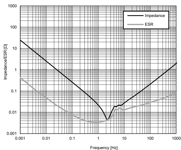
⑥2012X7SB106KS
