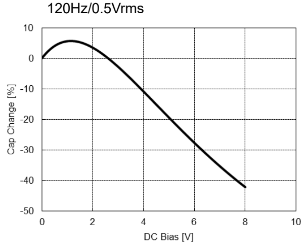
⑥2012X7SB106KS
