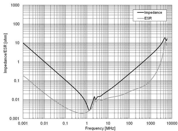
⑥2012X7SB106KS
