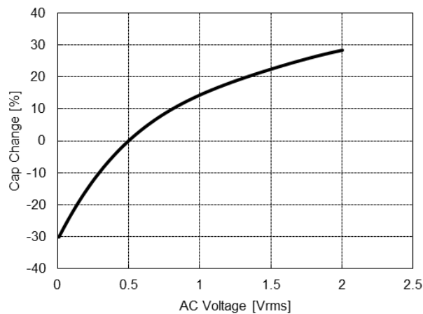
⑥2012X7SB106KS
