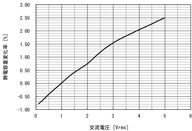
⑪N2040/L104-5750X7R2H104K
