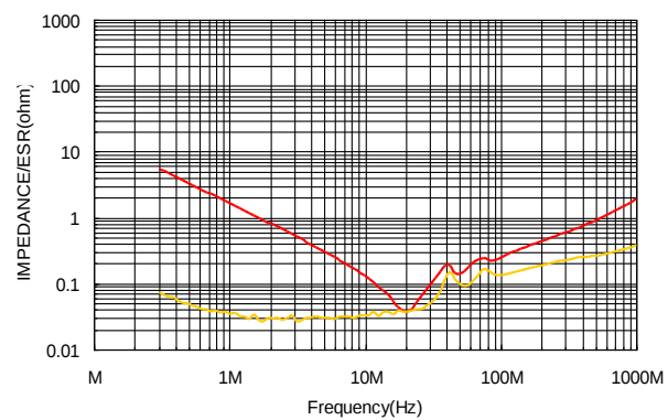
⑪N2040/L104-5750X7R2H104K
