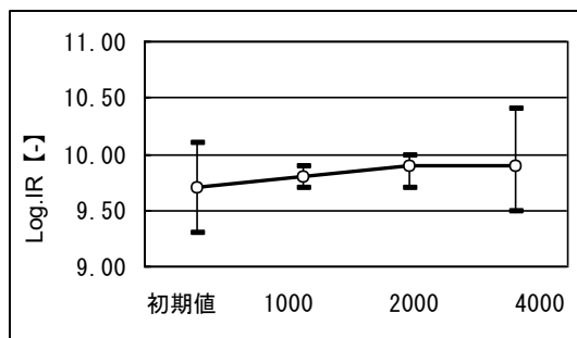
IR 常温 (25°C)
