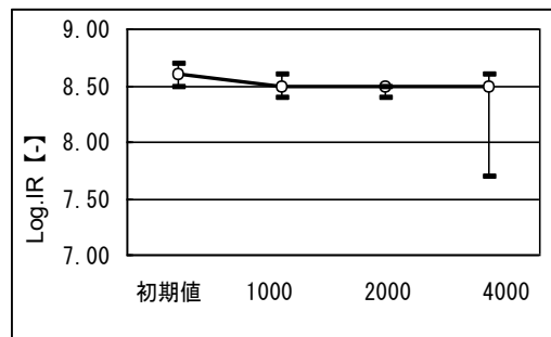
IR 高温時 (125°C)
