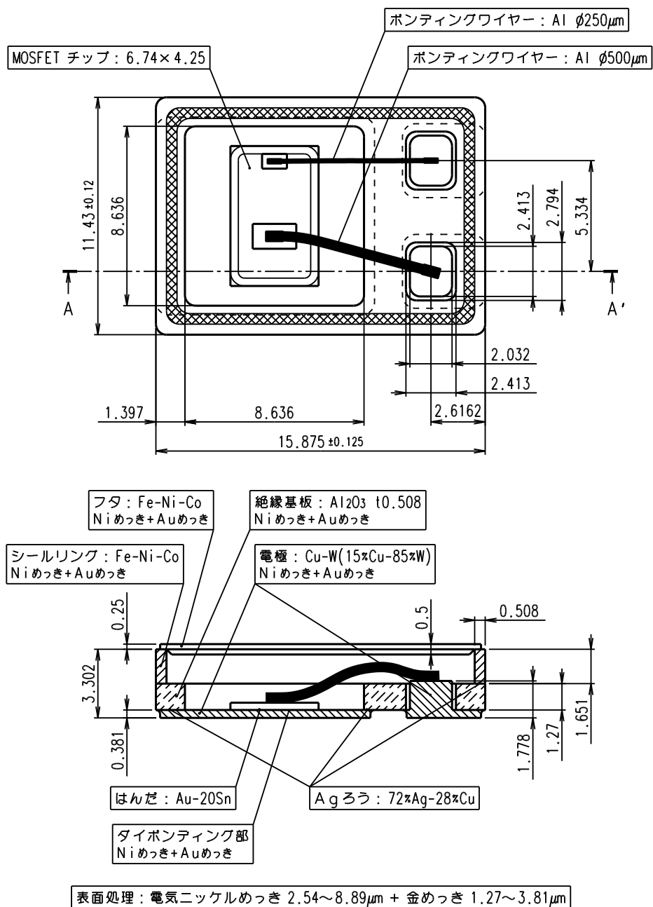
A-A' 断面図
