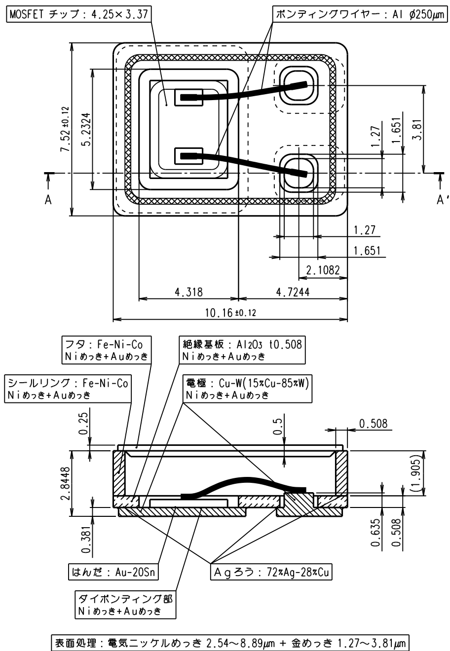
A-A' 断面図
