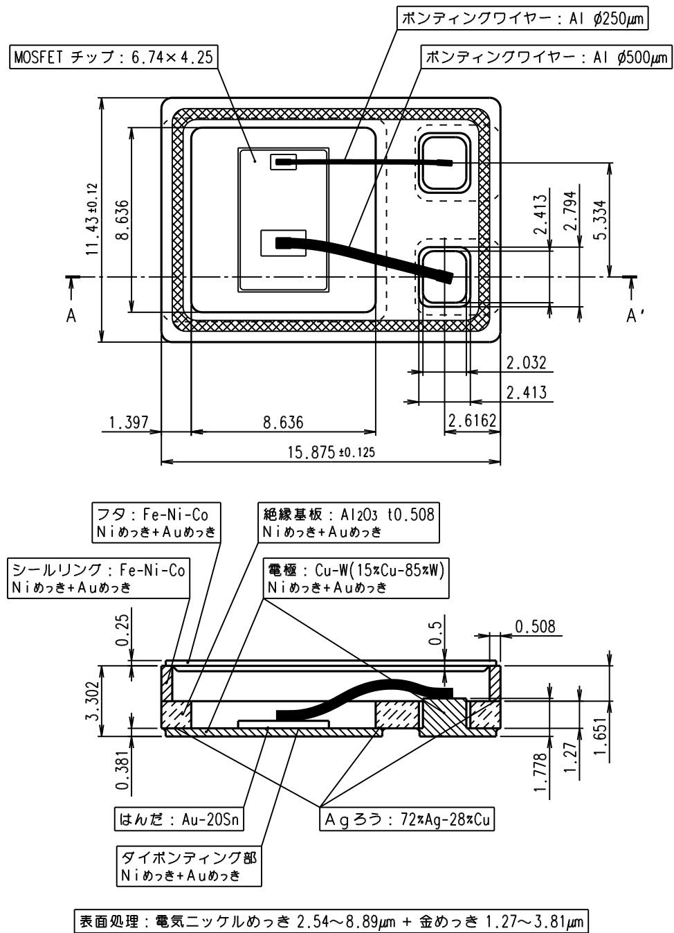
A-A' 断面図
