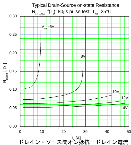
図 39 特性曲線 JAXA R 2SK4219 (1/3)
