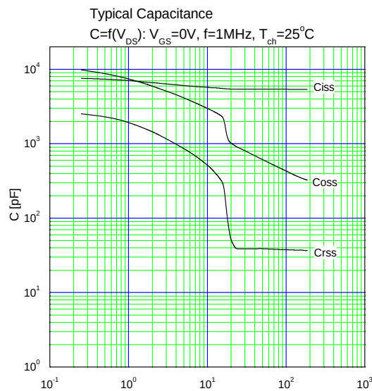
容量ードレイン・ソース間電圧
