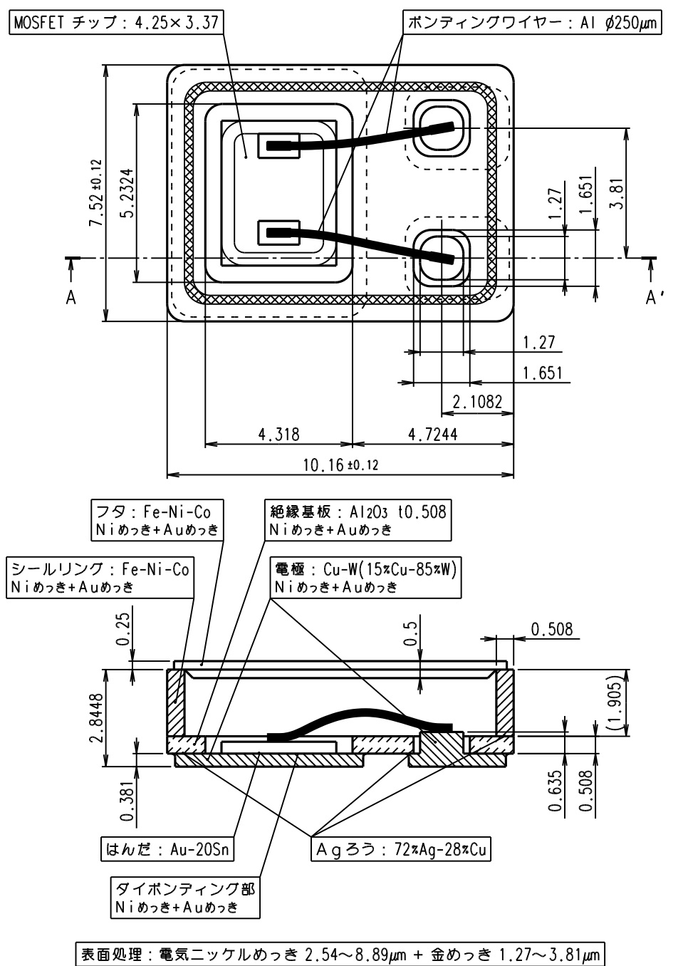
A-A' 断面図
