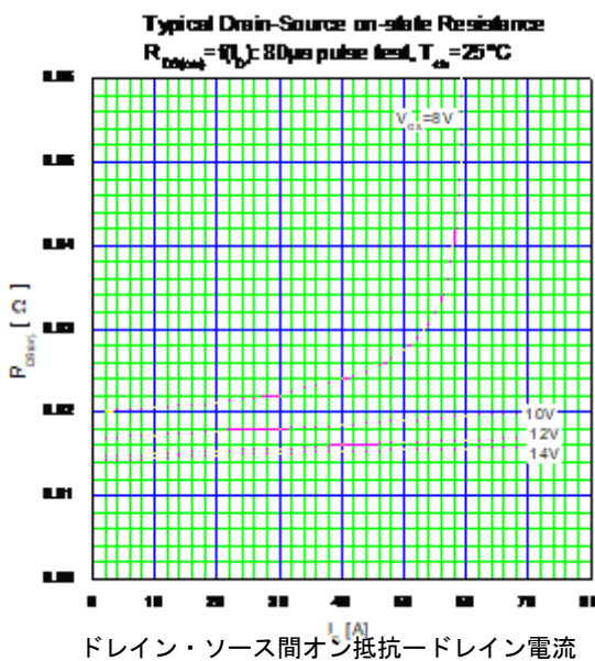
図 6 特性曲線 JAXA R 2SK4152 (1/3)
