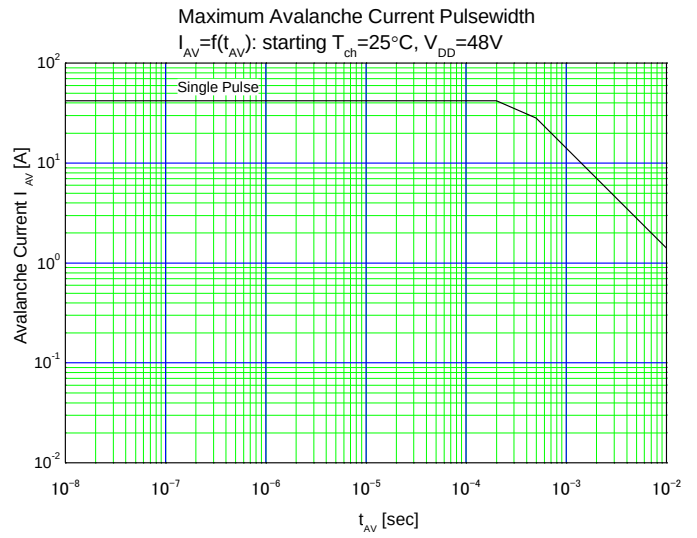
図 8 特性曲線 JAXA R 2SK4152 (3/3)
