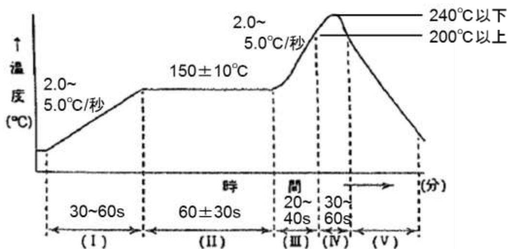
図 A 推奨リフロー温度プロファイル
