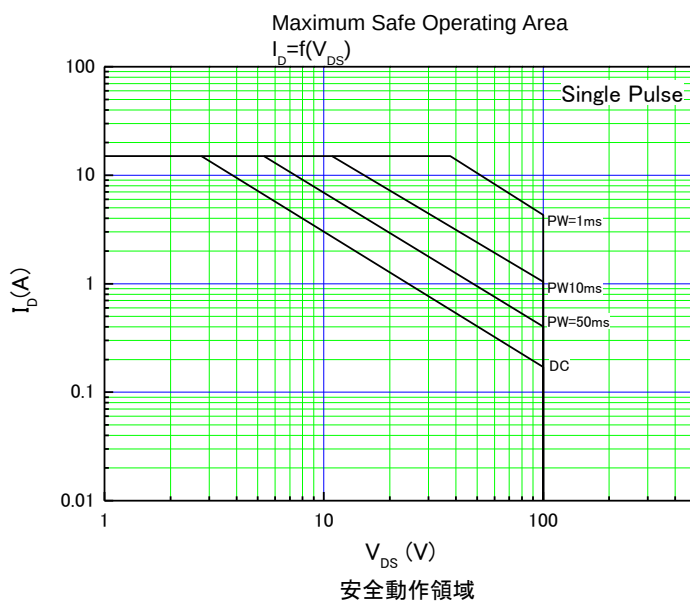
図 40 特性曲線 JAXA R 2SK4219 (2/3)
