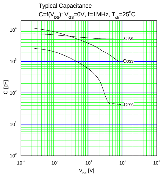
容量ードレイン・ソース間電圧
