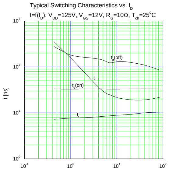
スイッチング時間ードレイン電流
